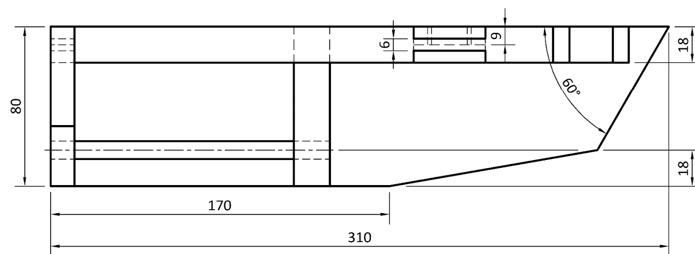
Plan/Bonnchló
