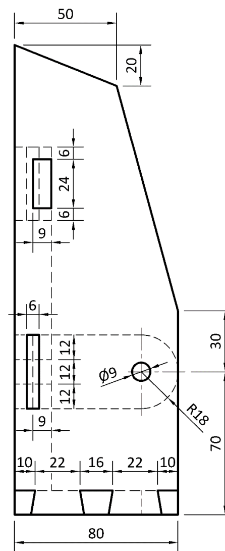
End View/Taobhchló
